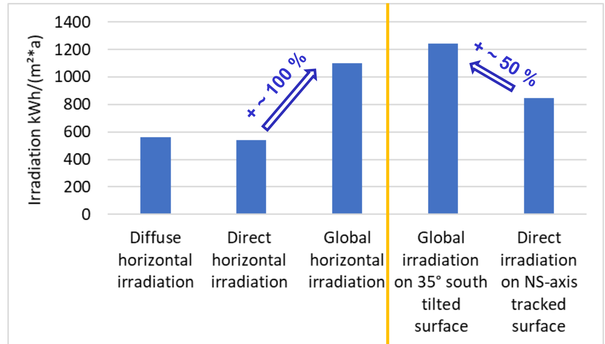
Jahressummen der Einstrahlung für den Standort Würzburg
